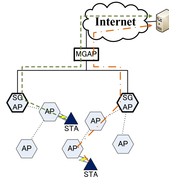
図2 GWの二重化
