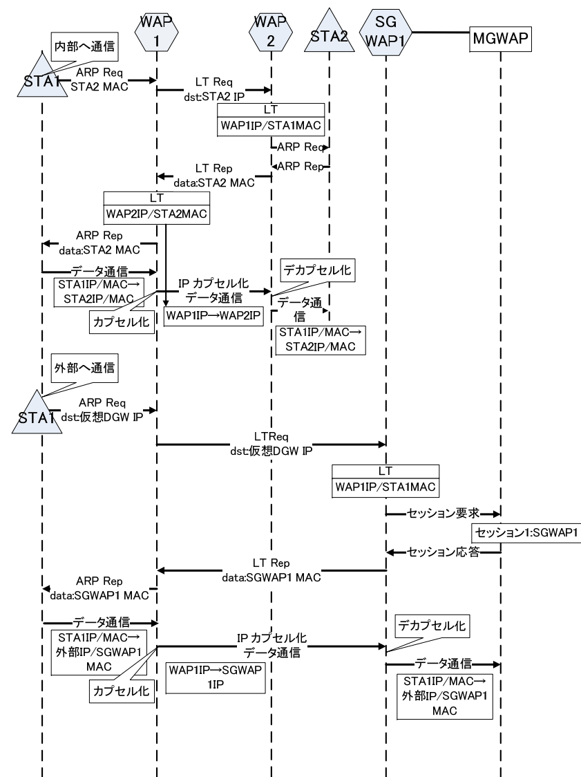
図 4 提案システム動作シーケンス
