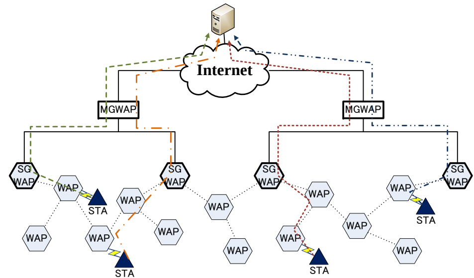
図 3 提案システム概要
