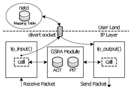
図 6 GSRA ルータの実装
