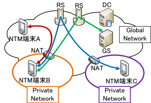
図 4 NTMobile のネットワーク構成
