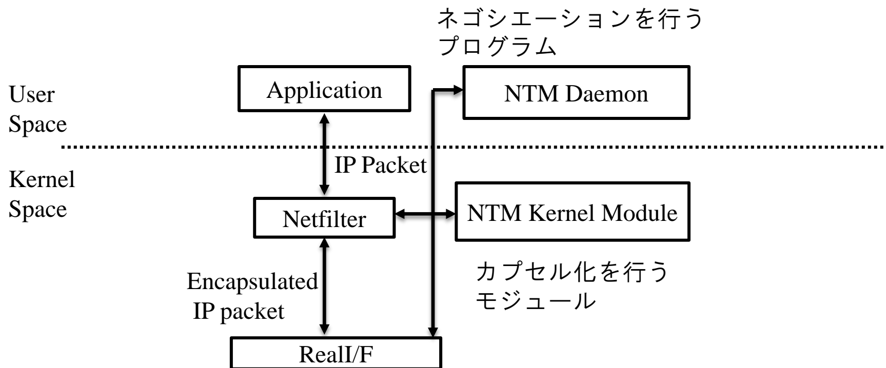
NTM端末のモジュール構造
