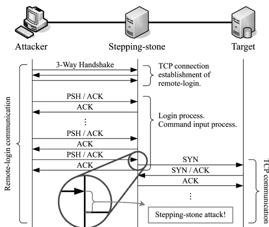
図 4 コネクションベース方式の原理 Fig. 4 The principle of Connection Base Method.
