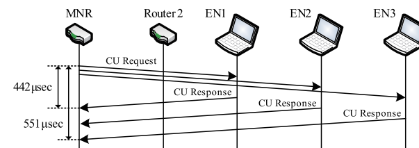
図 13 Mobile NPC のアドレス通知時間
