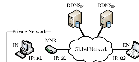
図3 Mobile NPC のネットワーク構成
