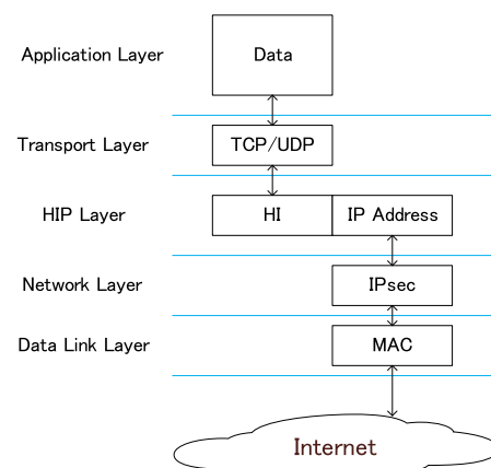
図 4 HIP のレイヤーモデル Fig. 4 Layer model of HIP.
