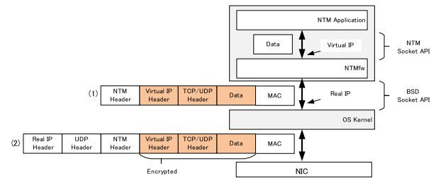
図 6 NTMfw のカプセル化通信の実現方法
