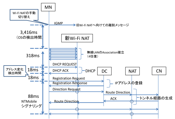
図 11 移動処理の試験結果
