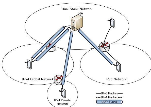
図 3 DSMIPv6 の構成 Fig. 3 Configuration of DSMIPv6.
