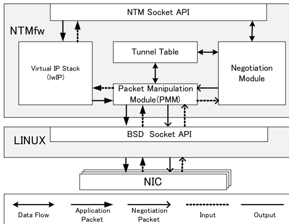
図 7 NTMfw のモジュール構成
