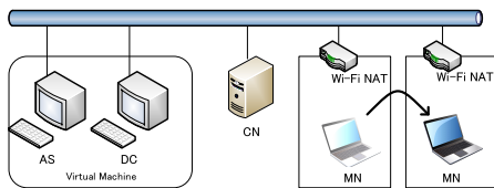
図 10 実験ネットワークの構成
