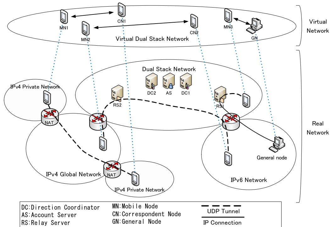
図 5 NTMobile の概要
